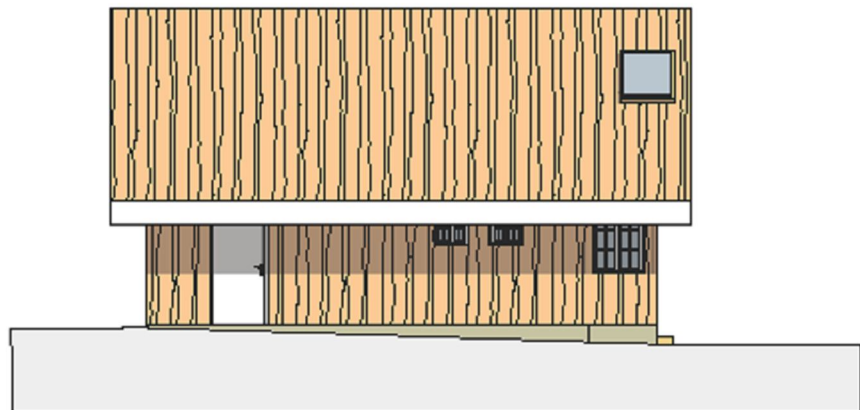
1:100 Fasade Nord
